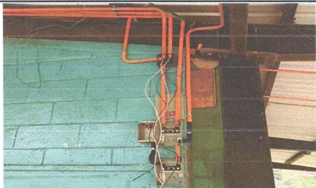
Foto 1: SUSTITUCIÓN DE SISTEMA ELECTRICO Y SUS ACC ESORIOS
